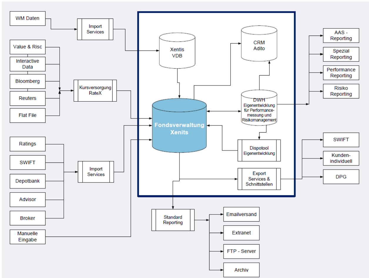
Abbildung 6: BayernInvest IT-Architektur
